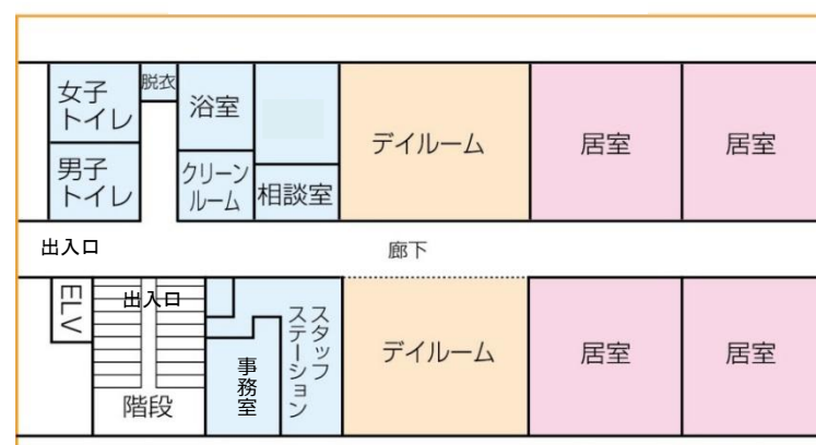
ことぶきの家 平面図
